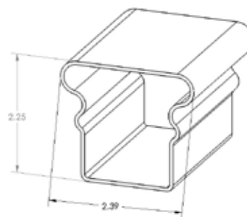
1-3/4" NEXUS® 2 T-RAIL
