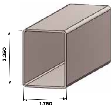
1-3/4" X 2-1/4" NEXUS®
